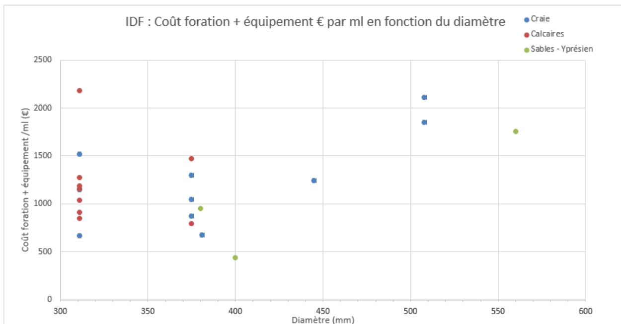
Figure 14 Coût additionné des postes de foration et équipement par mètre linéaire de forage en fonction du diamètre de foration et de la géologie pour la réalisation d'un forage de reconnaissance (opérations situées en Ile-de-France).
