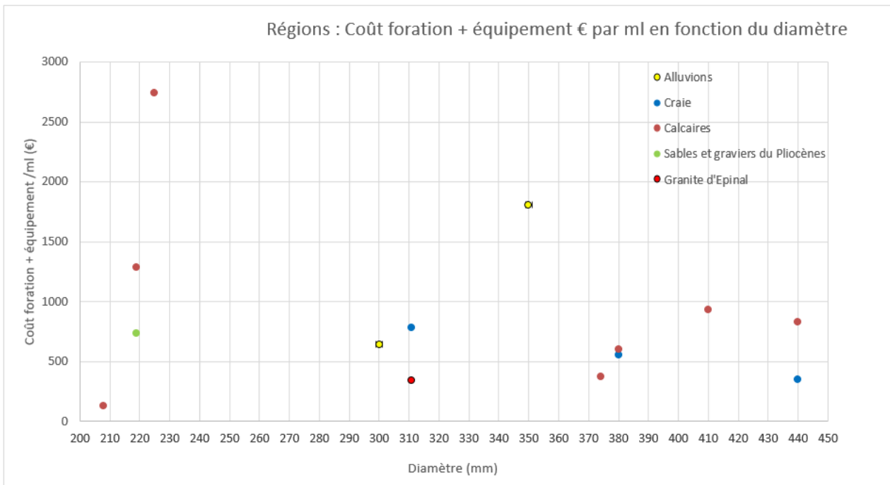
Figure 15 Coût additionné des postes de foration et équipement par mètre linéaire de forage en fonction du diamètre de foration et de la géologie pour la réalisation d'un forage de reconnaissance (opérations situées hors Ile-de-France).
