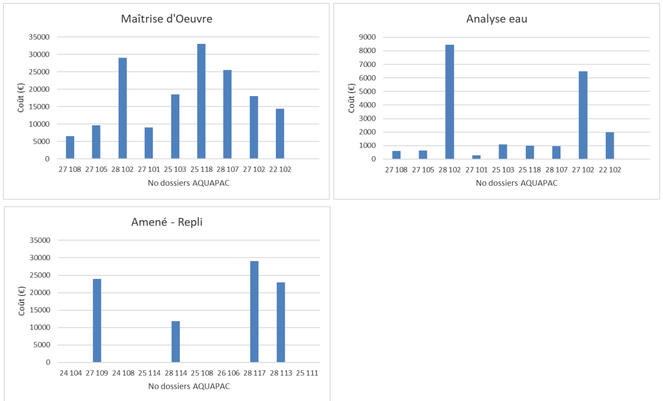
Figure 21 Mise en relation du coût du poste « maîtrise d'oeuvre » avec la profondeur pour des opérations situées en Ile-de-France dans la craie . Représentation sous la forme d'histogrammes du coût des postes « maîtrise d'oeuvre », « amenée – repli » et « analyse d'eau ».
