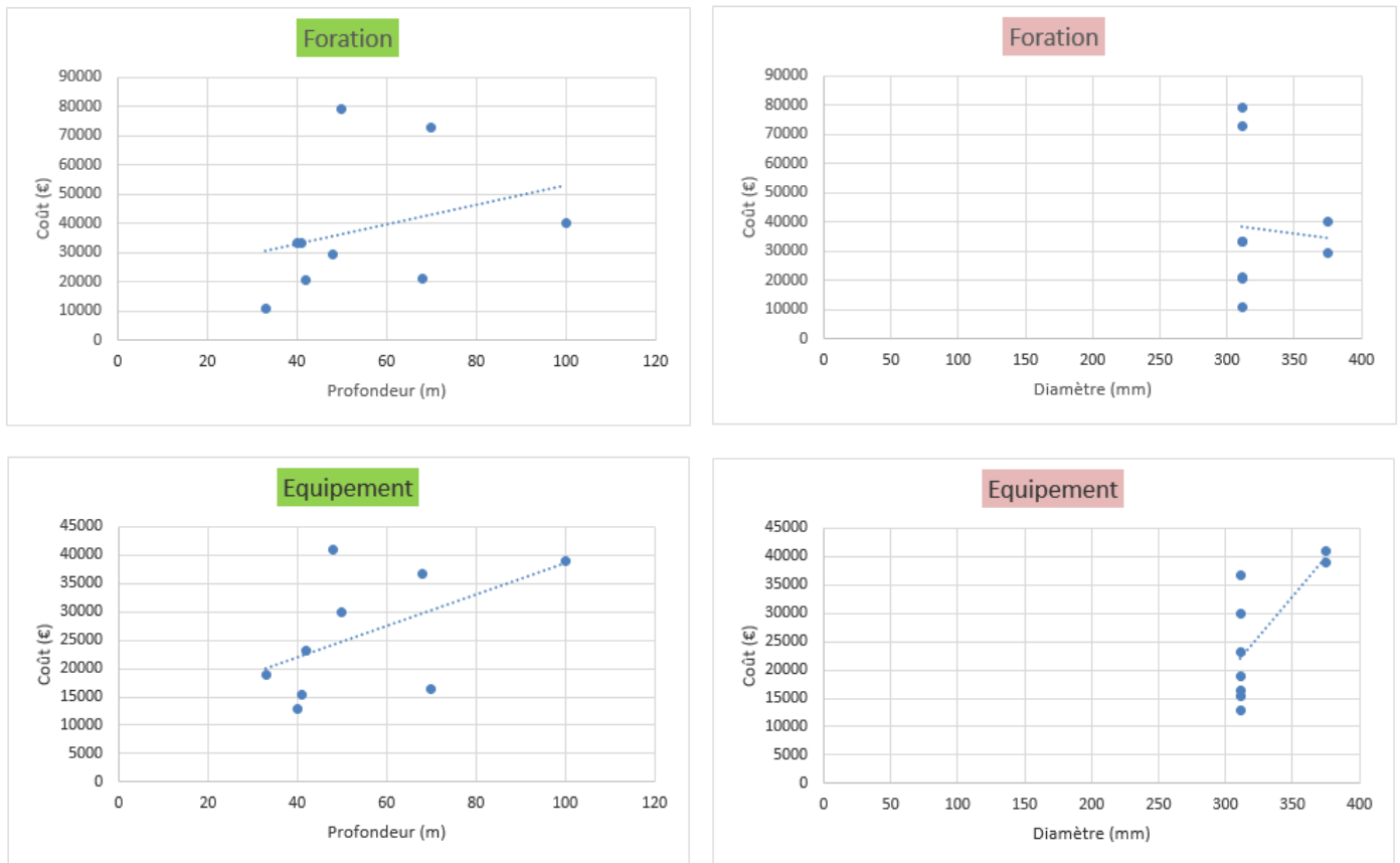
Figure 19 Mise en relation du coût des postes de « foration » et « d'équipement » avec la profondeur (à gauche) et le diamètre (à droite) pour des opérations situées en Ile-de-France dans les calcaires . L'objectif de dégager une courbe de tendance linéaire représentative (surligné en vert).
