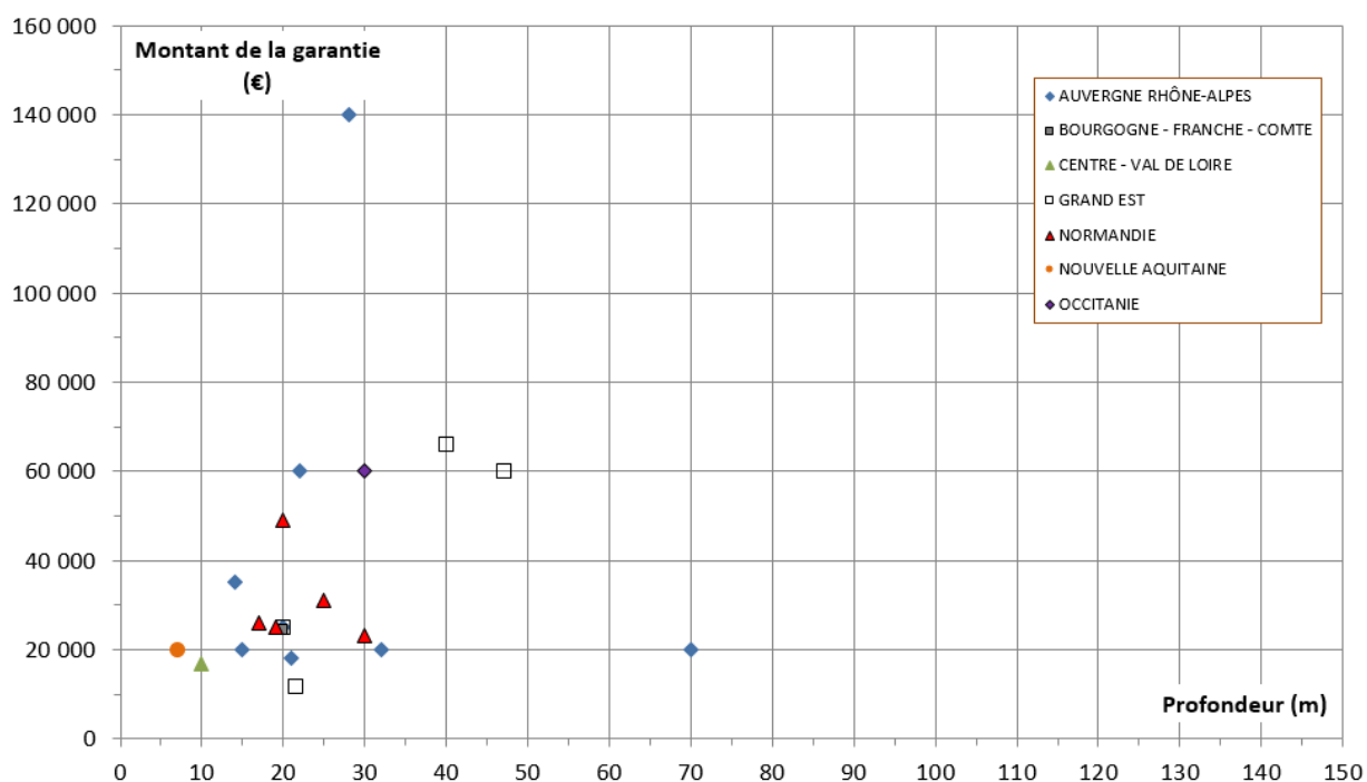
Figure 5 Répartition régionale des montants de garantie en fonction de la profondeur pour la réalisation d'un forage de reconnaissance dans les alluvions
