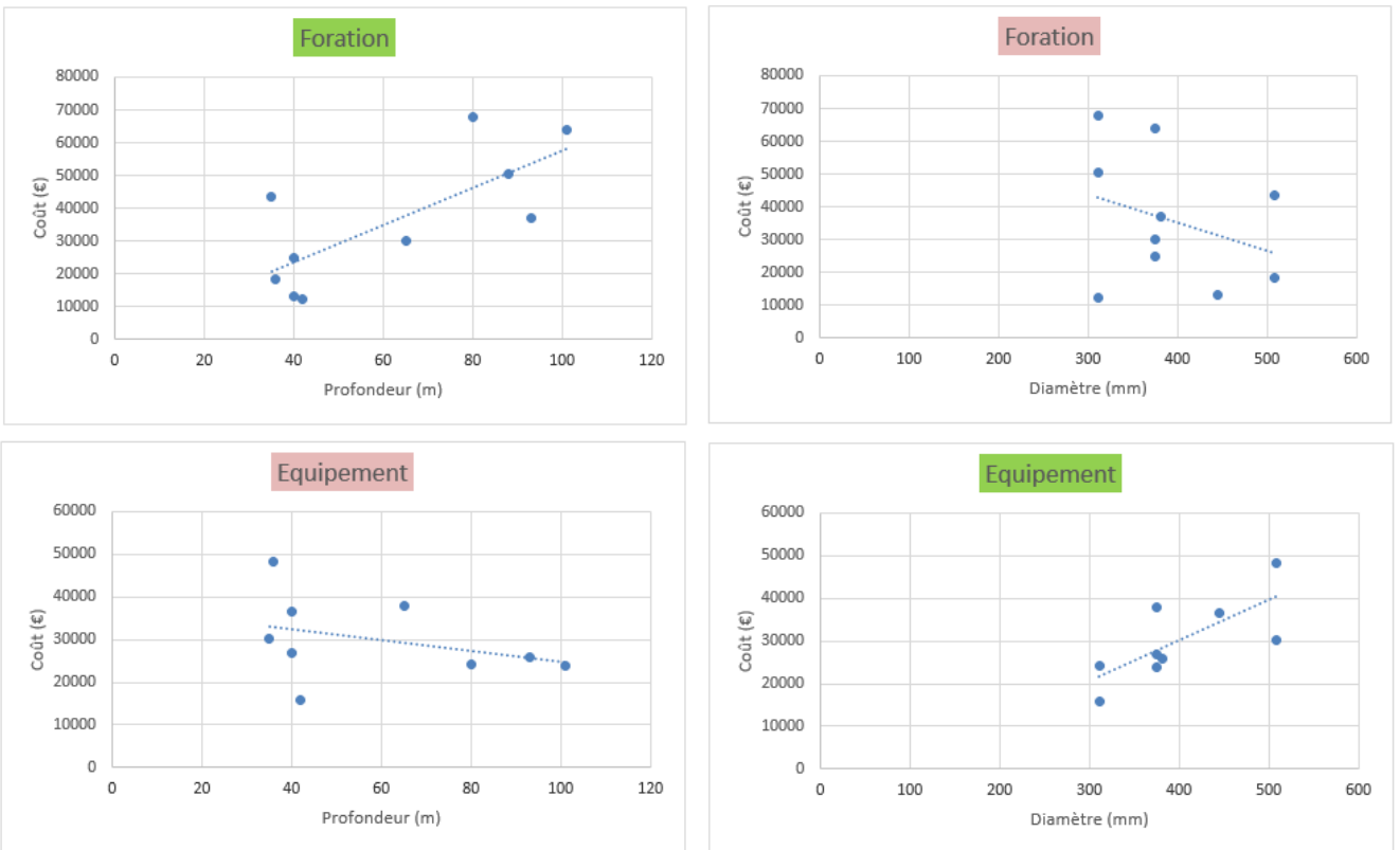
Figure 16 Mise en relation du coût des postes de « foration » et « d'équipement » avec la profondeur (à gauche) et le diamètre (à droite) pour des opérations situées en Ile-de-France dans la craie. (l'objectif de dégager une courbe de tendance linéaire représentative est surligné en vert).
