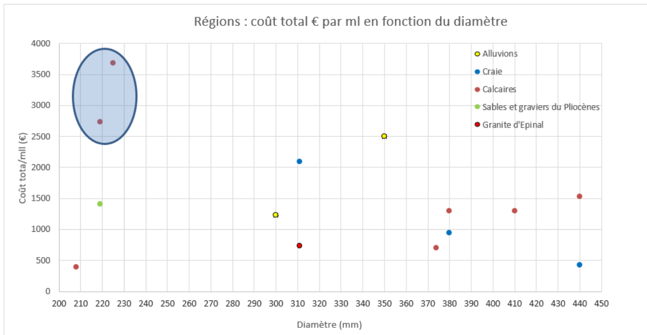
Figure 13 Coût total par mètre linéaire de forage en fonction du diamètre de foration et de la géologie pour la réalisation d'un forage de reconnaissance (opérations situées hors Ile-de-France). Les opérations situées dans le cercle bleu présentent un coût total anormalement élevé.
