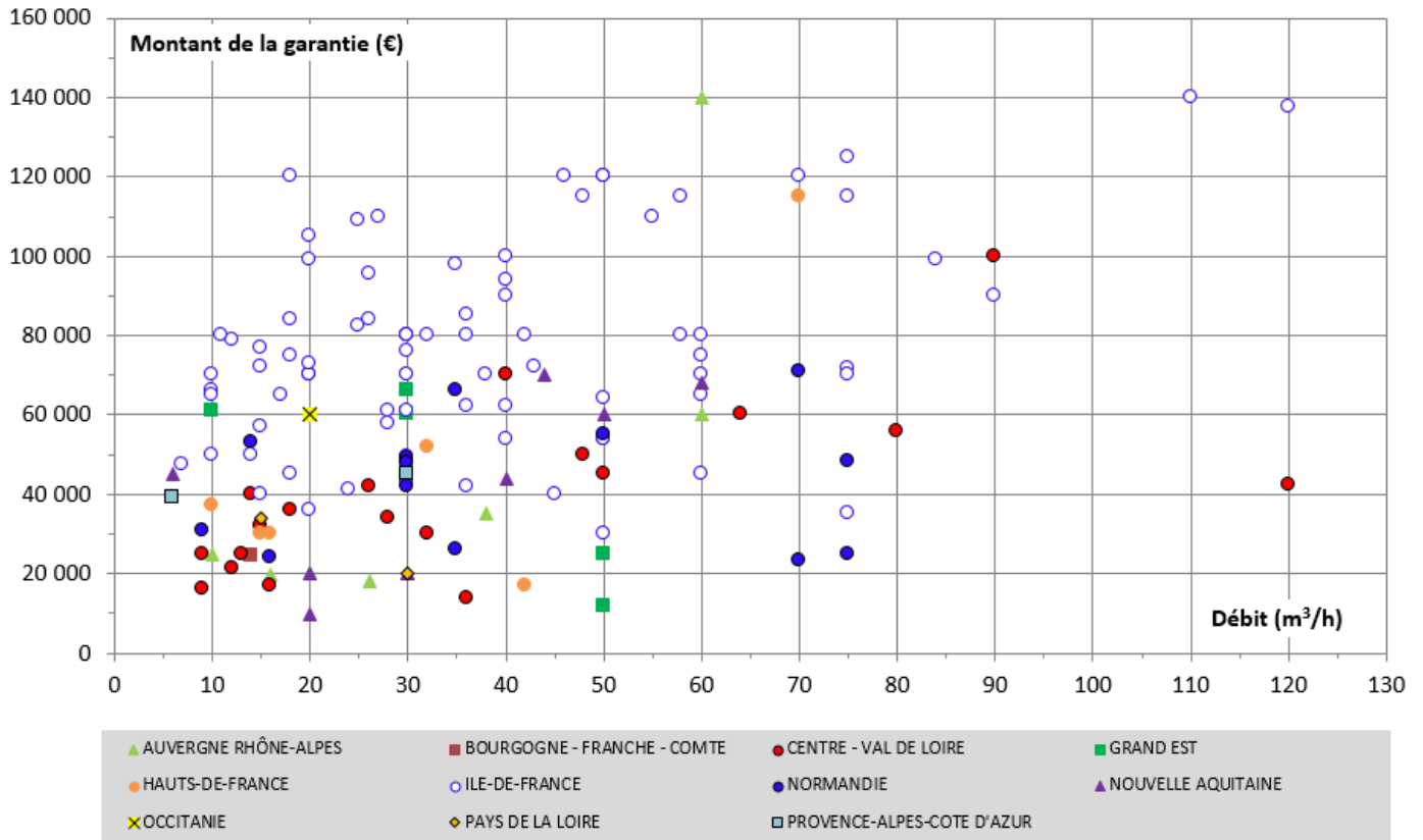
Figure 11 Répartition par région des montants de garantie pour la réalisation d'un forage de reconnaissance en fonction du débit (période 2014 – 2019)
