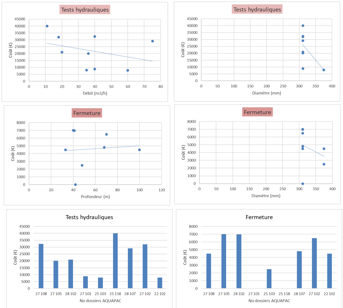
Figure 20 Mise en relation du coût du poste « tests hydrauliques » avec le débit (à gauche) et le diamètre (à droite), « fermeture » avec la profondeur (à gauche) et le diamètre (à droite) pour des opérations situées en Ile-de-France dans les calcaires . L'objectif de dégager une courbe de tendance linéaire représentative (surligné en vert). Aucune relation représentative entre le coût de la fermeture et la profondeur ou le diamètre n'a pû être dégagée. Représentation sous la forme d'histogramme du coût des postes « tests hydrauliques » et « fermeture ».
