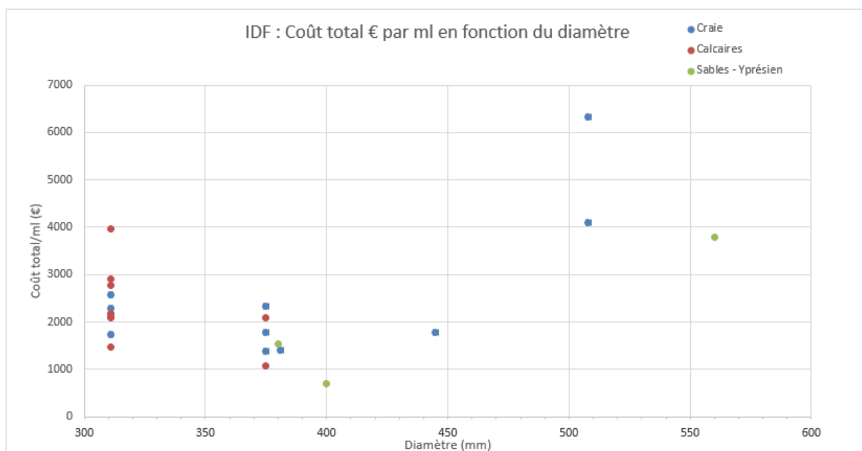
Figure 12 Coût total par mètre linéaire de forage en fonction du diamètre de foration et dans la craie, les calcaires et les sables de l'Yprésien pour la réalisation d'un forage de reconnaissance (22 opérations situées en Ile-de-France).
