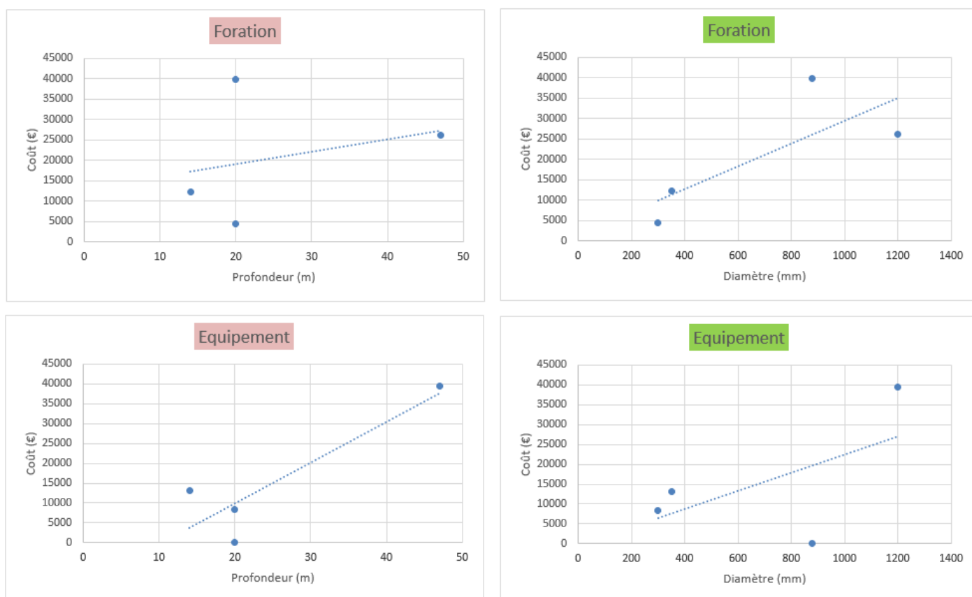
Figure 22 Mise en relation du coût des postes de « foration » et « d'équipement » avec la profondeur (à gauche) et le diamètre (à droite) pour des opérations situées hors Ile-de-France dans les alluvions . Les courbes de tendance linéaire sont données à titre indicatif en raison du nombre de données trop faible. Les relations représentatives ont été surlignées en vert.
