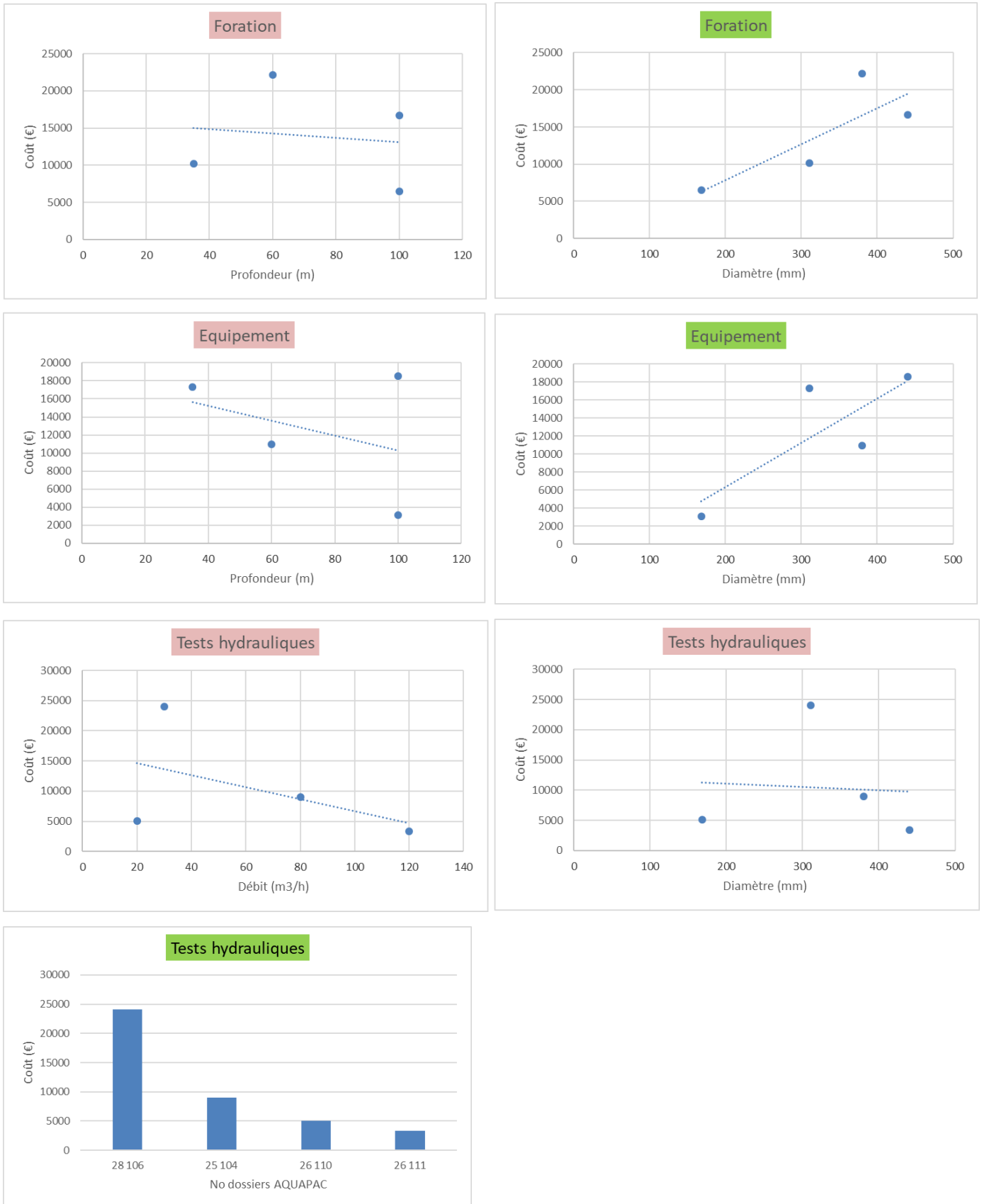
Figure 25 Mise en relation du coût des postes de « foration » et « d'équipement » avec la profondeur (à gauche) et le diamètre (à droite) pour des opérations situées hors Ile-de-France dans la craie . Aucune relation représentative entre le coût des tests hydrauliques et la profondeur ou le diamètre
