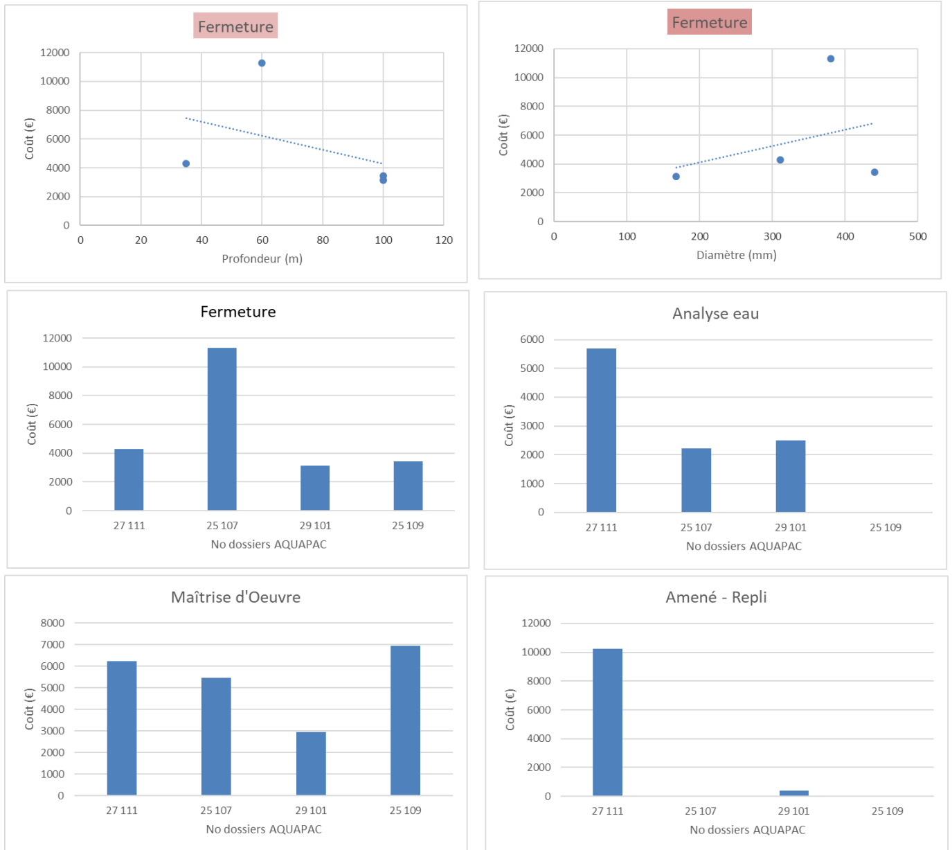
Figure 26 Mise en relation du coût du poste « fermeture » avec la profondeur (à gauche) et le diamètre (à droite) pour des opérations situées dans les régions hors Ile-de-France dans la craie . Aucune relation représentative entre le coût de la fermeture et la profondeur ou le diamètre n'a pû être dégagée. Représentation sous la forme d'histogramme du coût des postes « fermeture », « analyse d'eau », « maîtrise d'oeuvre » et « amenée - repli ».
