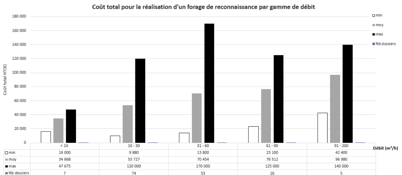
Figure 10 Montant garanti (coûts totaux minimum, moyens, maximum) par gamme de débits (m 3 /h)
