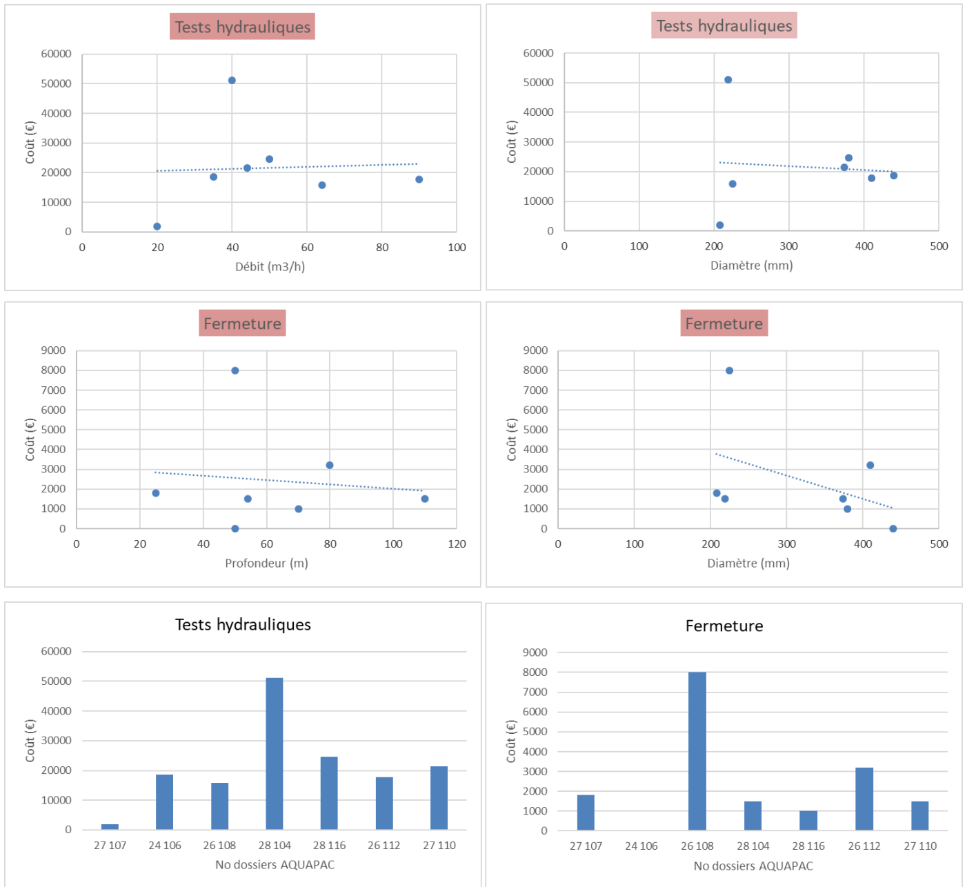
Figure 28 Mise en relation du coût du poste « tests hydrauliques » avec le débit (à gauche) et le diamètre (à droite), « fermeture » avec la profondeur (à gauche) et le diamètre (à droite) pour des opérations situées dans les régions hors Ile-de-France dans les calcaires . Aucune relation représentative n'a pu être dégagée pour ces deux postes. Représentation sous la forme d'histogrammes du coût des postes « tests hydraulique » et « fermeture ».
